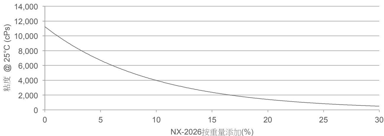
NX-2026与液体环氧树脂混合的稀释曲线图（环氧当量=190
